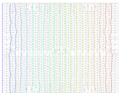
Figura 2 - Mesh dell'elemento ed andamento delle isoterme.
